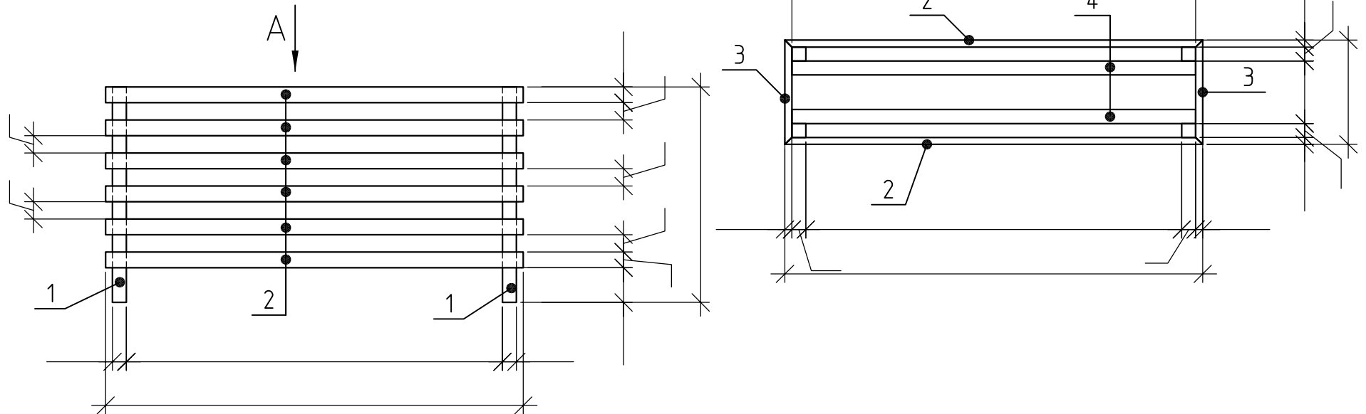
Схема расположения конструкций кашпо
